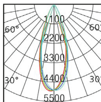
30W 3000K 36deg
