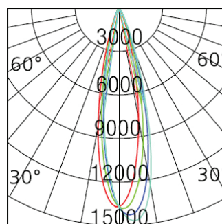
L646 3000K 24deg
